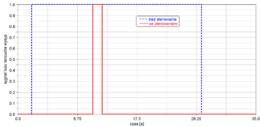
Rys. 7. Wartości sygnału z przetwornika detekcji stanu luzowania łańcucha na napędzie wysypowym, zarejestrowane podczas symulacji pracy przenośnika na upadzie [6]
