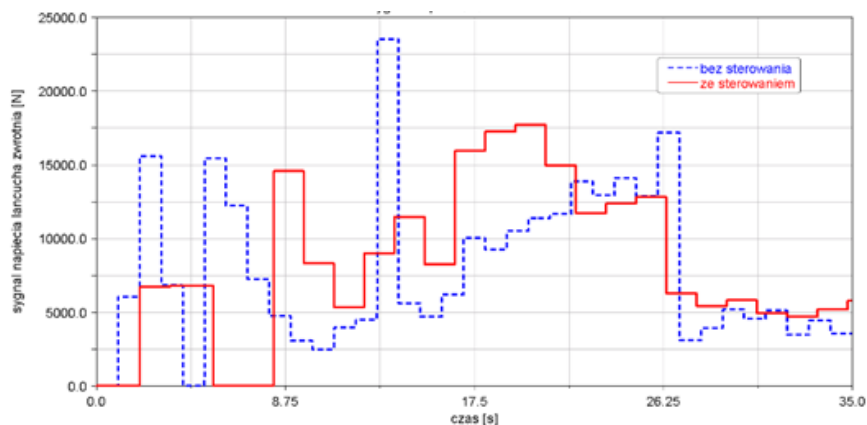
Rys. 5. Wartości siły nacisku zgrzebła na rynnę przenośnika na napędzie zwrotnym przenośnika, zarejestrowane podczas symulacji pracy przenośnika na upadzie [6]
